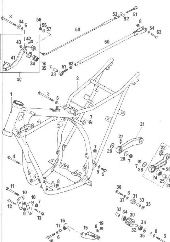
RAHMEN / Frame
